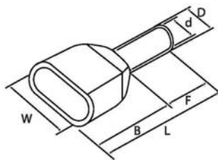
สลีปย้าปลายสายหุ้มฉนวนในลอนแบบคู่
